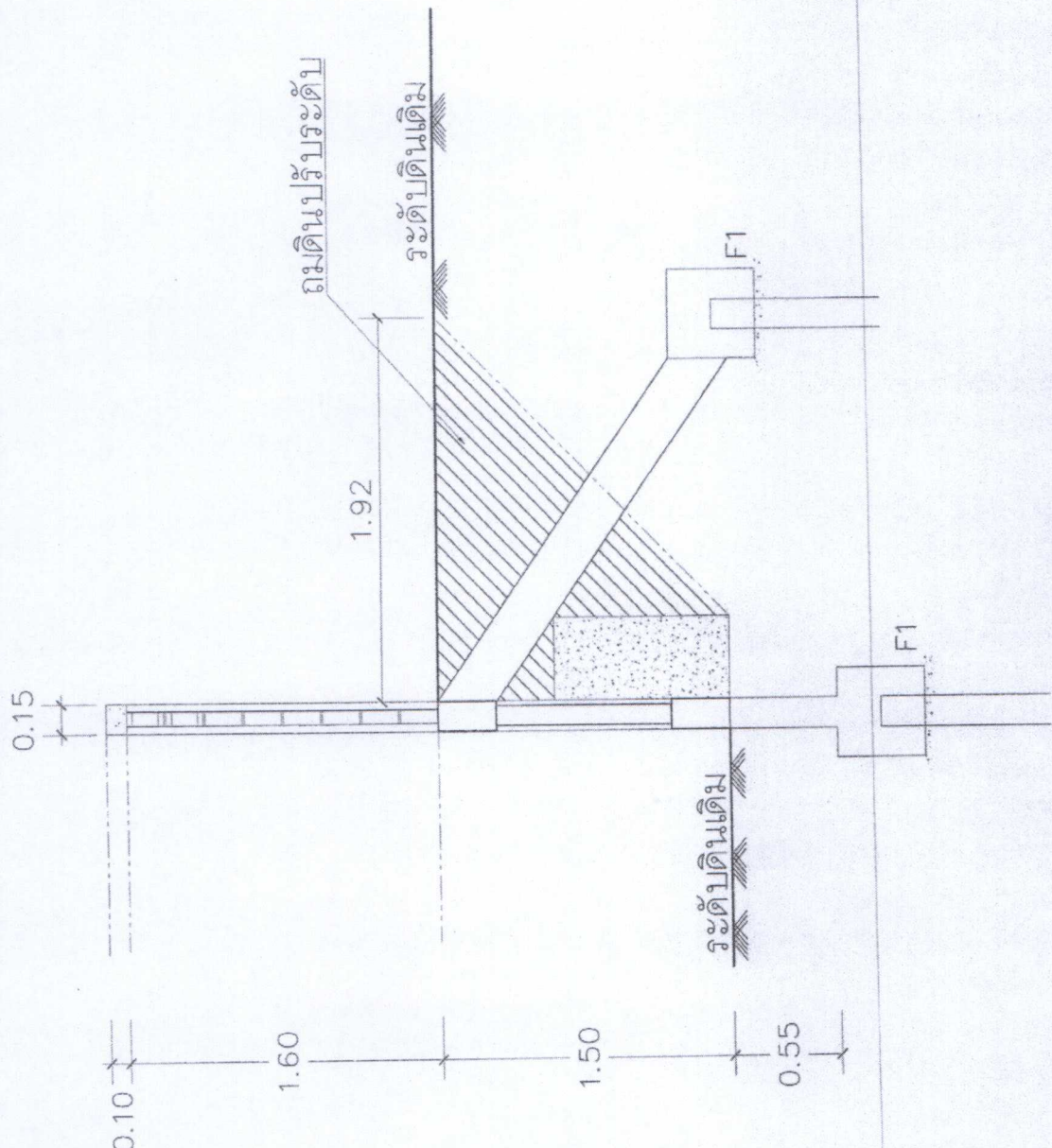
รูปตัดดินถม มาตราส่วน 1:50
